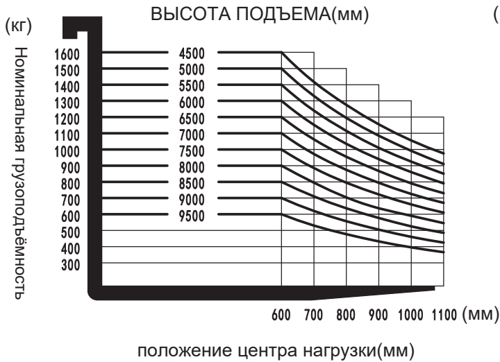
Диаграмма остаточной грузоподъемности
